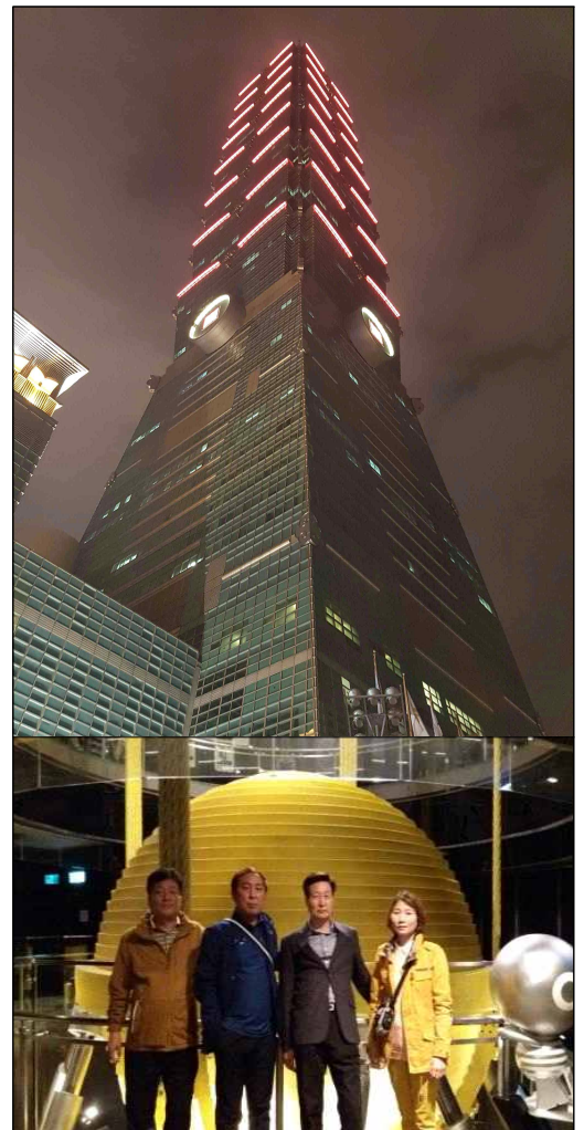
101빌딩의 상징 댐퍼, 지진이 발생하여 건물이 흔들리면 반대쪽으로 기울어 건물의 진폭을 줄여주는 내진설계 장치다. 이 댐퍼 덕분에 타이페이에 지진이 난다면 가장 안전한 곳이 101빌딩이라고 한다.
